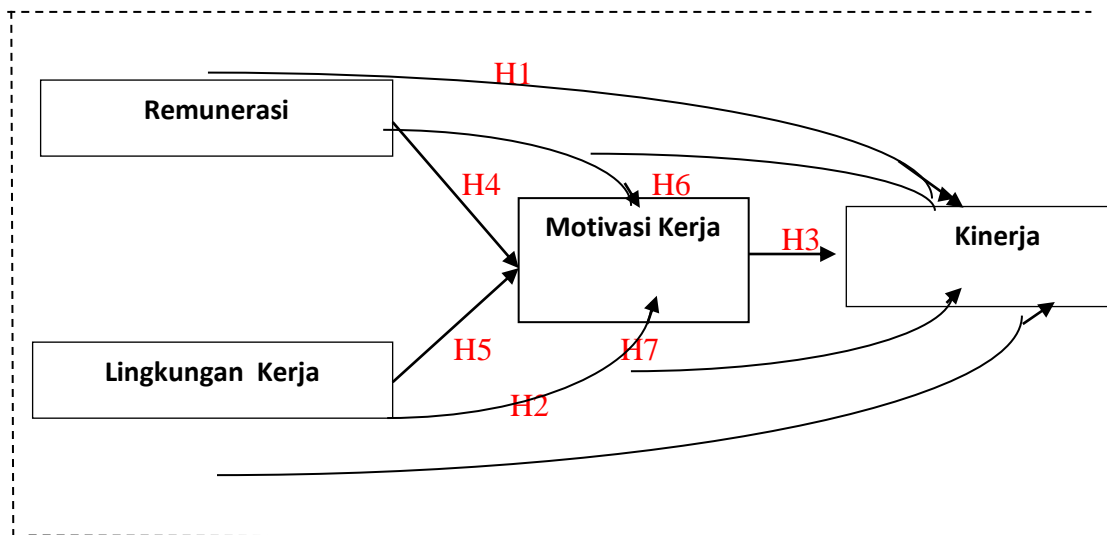
Gambar. 1 Kerangka Konsep
