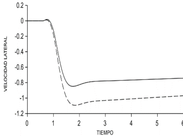
Figura 5 Velocidad lateral v_y (sólida) y v_{y,ref} (interlínea) [m/s vs s].
