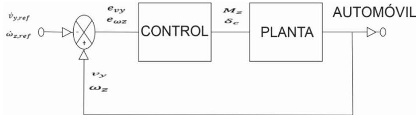
Figura 3 Diagrama a bloques del control por linealización-retroalimentación de estados.
