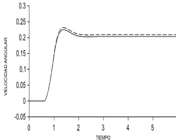
Figura 6 Velocidad angular de viraje \omega_z (sólida) y \omega_{z,ref} (interlínea) [rad/s vs s].
