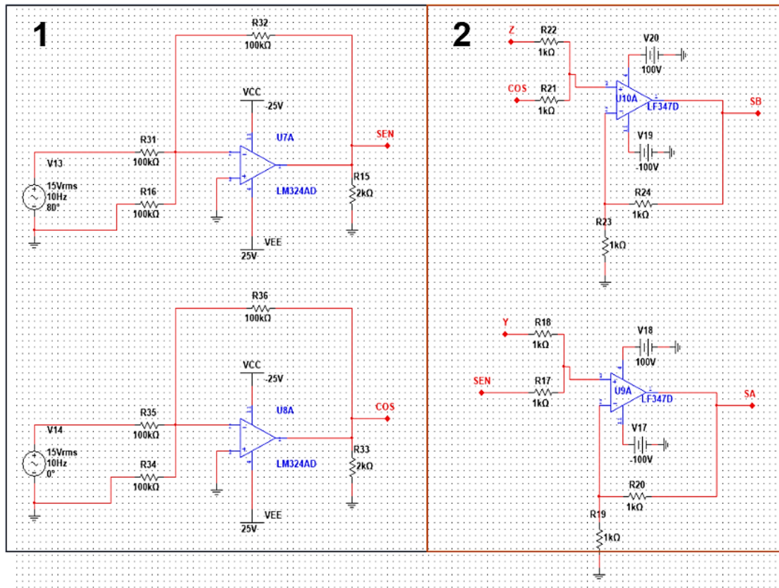
Figura 14 Circuito en NI Multisim para generar elipses.
