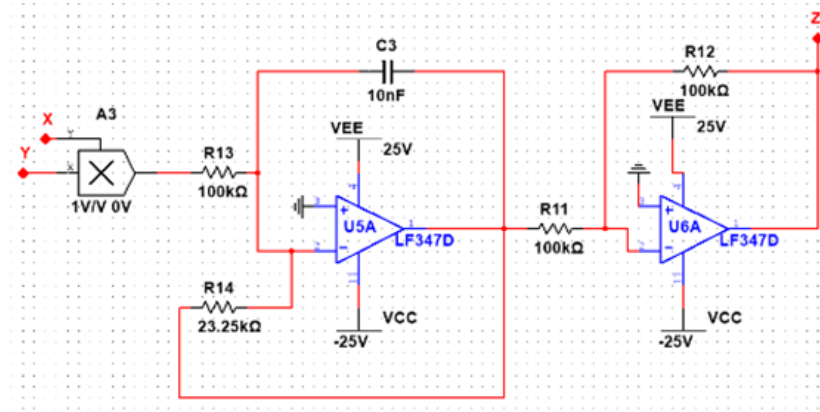
Figura 11 Diagrama esquemático de la expresión para la ecuación 13.
