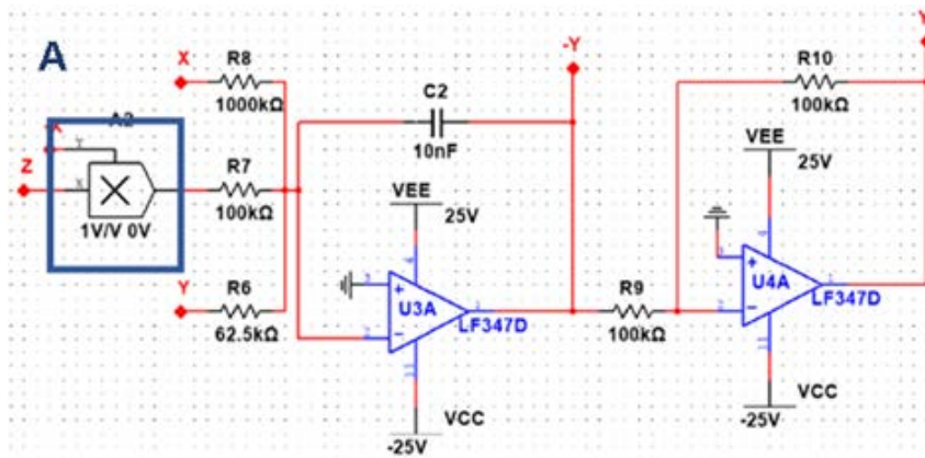
Figura 10 Circuito correspondiente a la ecuación 12.
