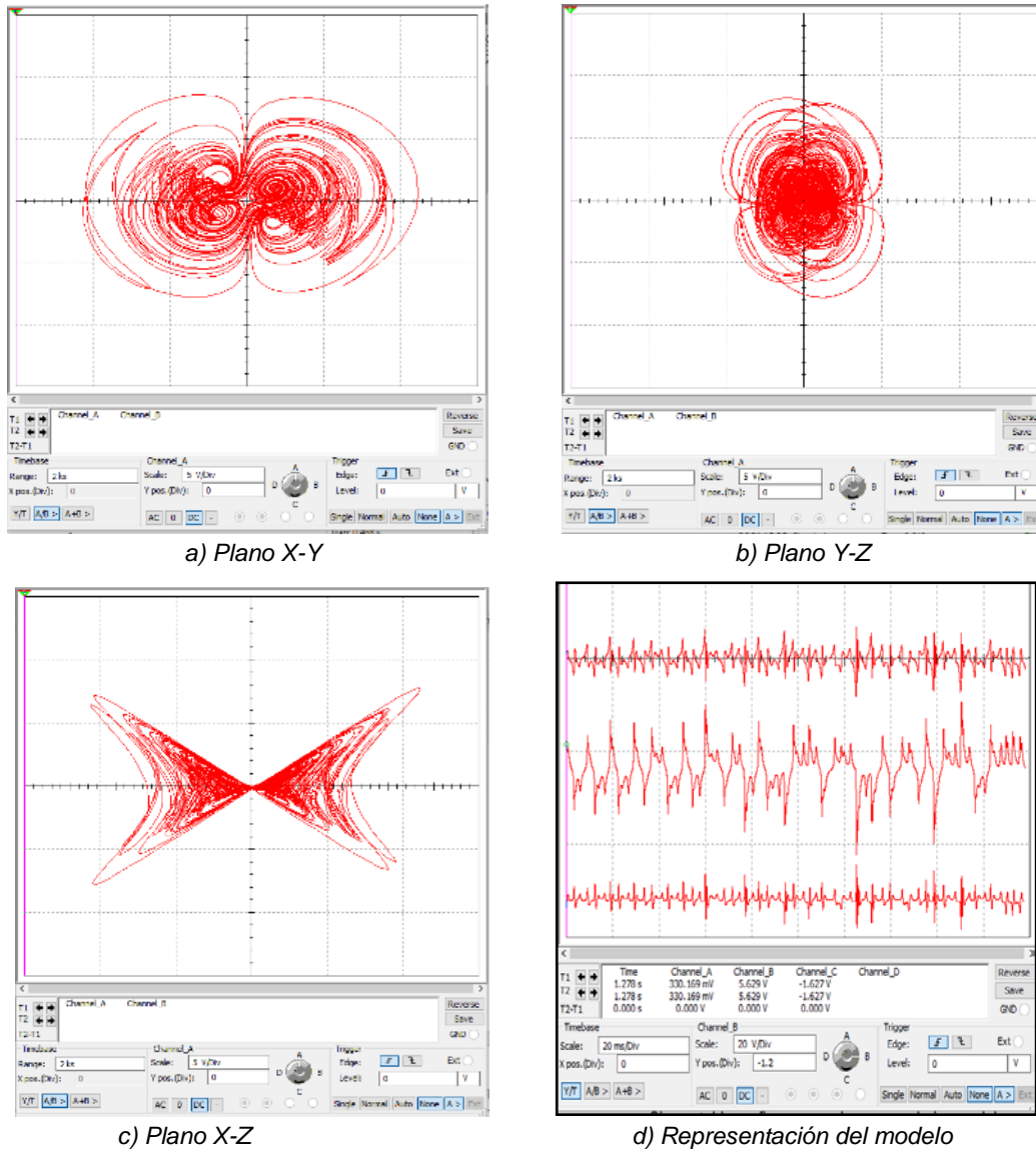
Figura 13 Modelo caótico del sistema en NI Multisim.
