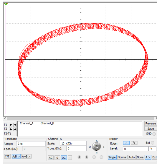
Figura 7 Caso 2, trayectoria caotica a lo largo de la orbita mostrando una configuración estable del sistema de cuatro alas.
