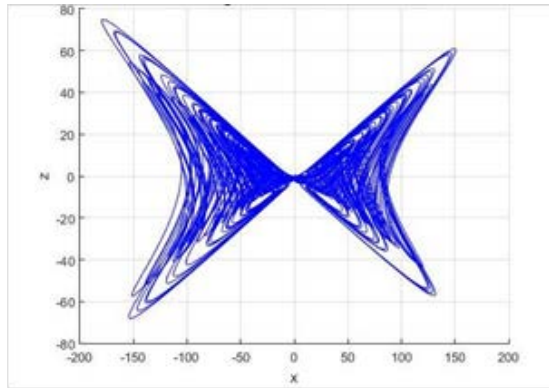
Figura 4 Sistema caótico de cuatro alas, plano Z-X.
