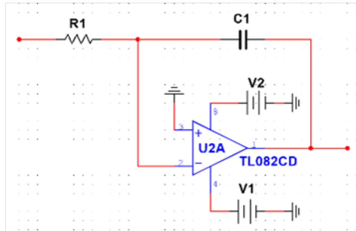
Figura 8 Principal arreglo utilizado para el sistema caótico de 4 alas, a este sistema se le agregan componentes para obtener las diversas combinaciones.
