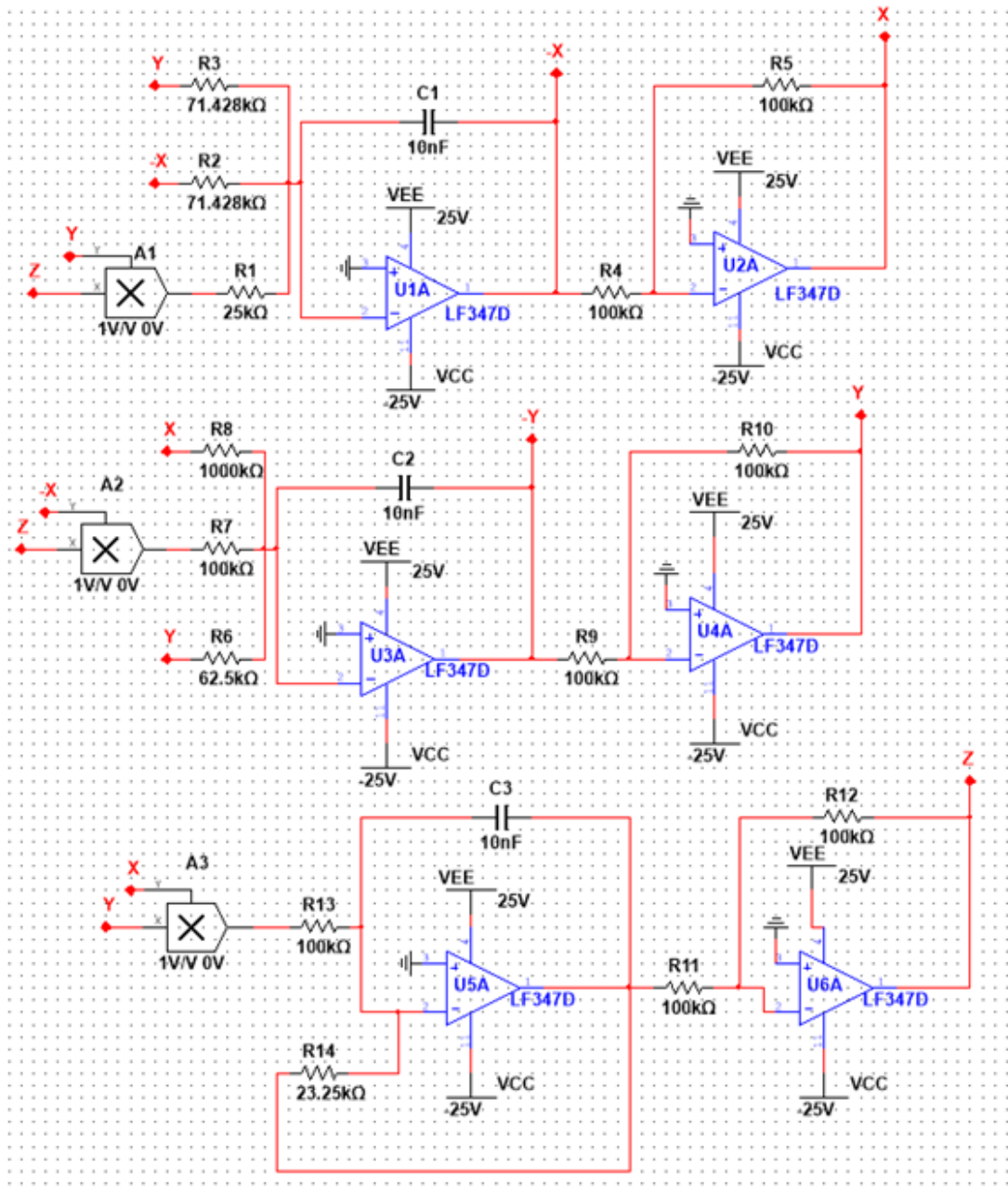
Figura 12 Circuito completo del sistema caótico de 4 alas para modelar el sistema.
