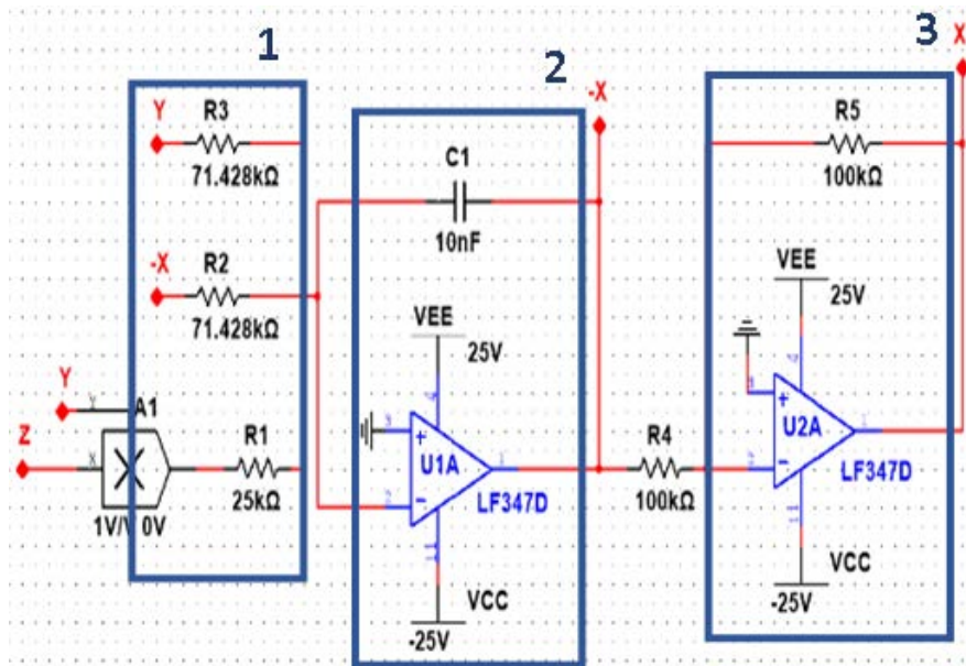
Figura 9 Esquema del circuito correspondiente a la ecuación (11).
