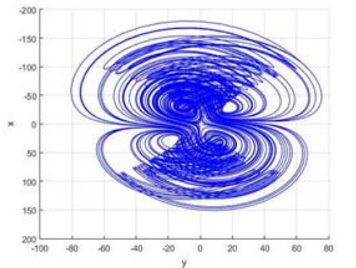
Figura 3 Sistema caótico de cuatro alas, plano X-Y.
