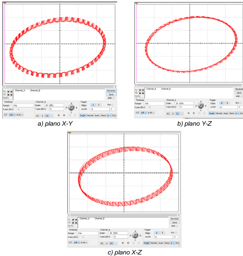
Figura 16 Trayectoria con caos correspondiente al CASO #2.
