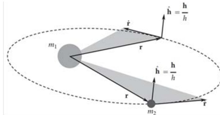
Figura 1 Diagrama del problema de los dos cuerpos.
