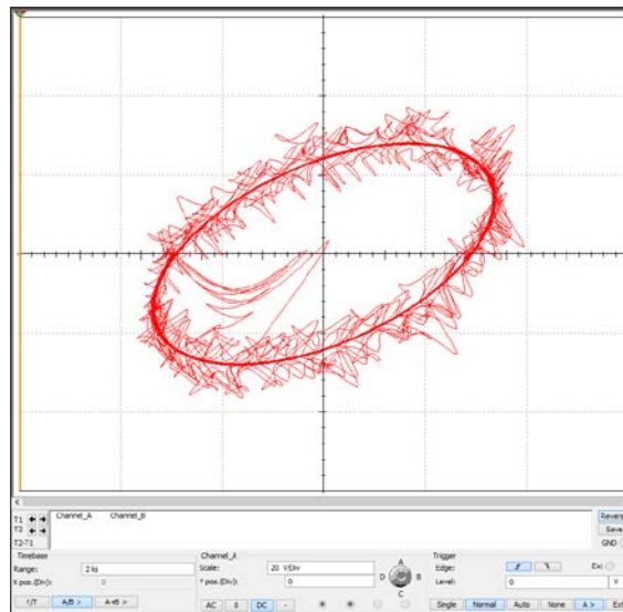
Figura 6 Caso 1, trayectoria caotica a lo largo de la orbita mostrando la inestabilidad del sistema de cuatro alas.
