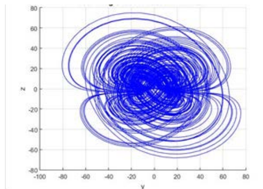
Figura 4 Sistema caótico de cuatro alas, plano Z-Y.
