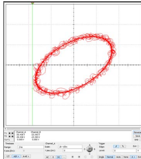
(b) Trayectoria con caos correspondiente al CASO #1
