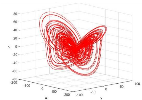
Figura 5 Sistema caótico de cuatro alas, plano X-Y-Z.
