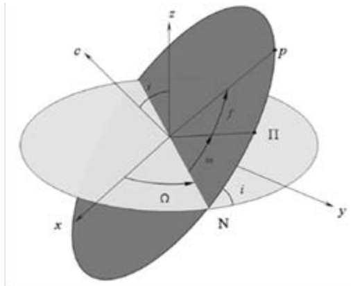
Figura 2 Definición de los ángulos de Euler.
