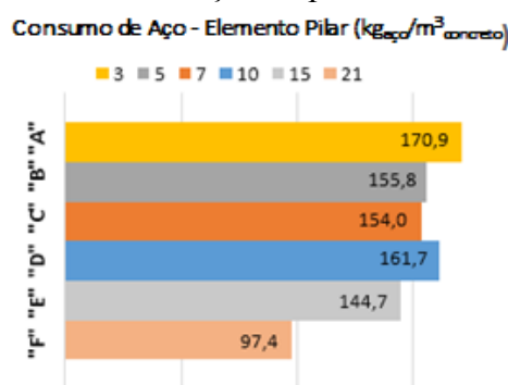
Figura 4: Consumo de aço dos pilares Casos “A até F”
