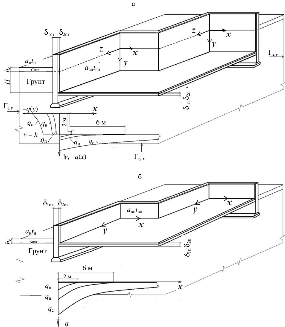
Рис. 1. Расчетная схема исследуемой области для зданий: а – заглубленного; б – незаглубленного; \delta_{1ст}, \delta_{2ст} \dots – толщина конструктивных слоев подземной части стены; \delta_{1л}, \delta_{2л} \dots – то же пола; \alpha_n, t_n – соответственно коэффициент теплообмена на наружной поверхности ограждения и текущее значение температуры наружного воздуха для расчетного периода; \alpha_{вн}, t_{вн} – то же на внутренней поверхности ограждения или пола и расчетная температура внутреннего воздуха; h_c – расчетная высота снежного покрова; H – глубина заложения поверхности пола по отношению к отметке поверхности земли
