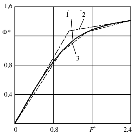
Рис. 1. 1 – кривая намагничивания тягового электродвигателя ДК-210А3; 2 – ее кусочно-линейная аппроксимация двумя отрезками касательных; 3 – то же тремя отрезками вписанной ломаной
