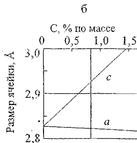
Рис. 5. Кристаллическая структура мартенсита: а – кристаллическая решетка; б – периоды решетки в зависимости от содержания углерода [3]
