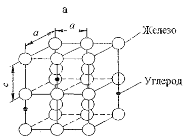
Рис. 5. Кристаллическая структура мартенсита: а – кристаллическая решетка; б – периоды решетки в зависимости от содержания углерода [3]
