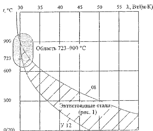
Рис. 4. Изменение теплопроводности эвтектидной стали (08; Ст. 1; Ст. 3; Ст. 5; Ст. 6; Ст. 7; Y 9; Y 10; Y 12; Y 13) при нагревании
