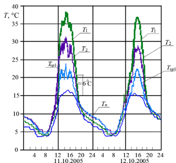
Рис. 1. Зависимости температур воздуха и поверхностей ограждения на юго-западной стороне книгохранилища библиотеки от времени суток за период 11–12 октября 2005 г.: T_n – температура наружного воздуха; T_1 – температура внутренней поверхности стекла; T_2 – температура наружной поверхности листа алюминия; T_{vp1} – температура воздуха между стеклом и алюминиевой стенкой на высоте 10 м от входа воздуха
