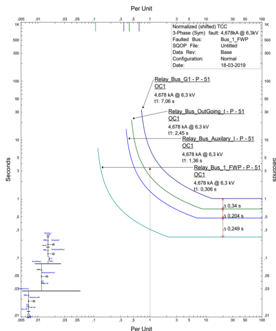
Gambar 4 Kurva Koordinasi Motor 1 FWP
