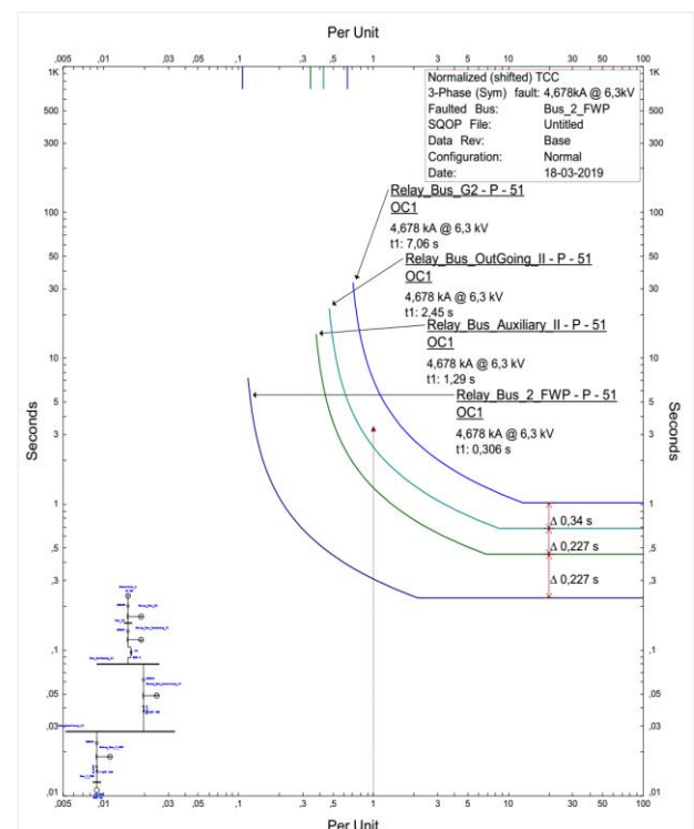
Gambar 6 Kurva Koordinasi Motor 2 FWP
