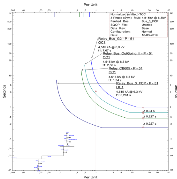
Gambar 7 Kurva Koordinasi Motor 3 FCP
