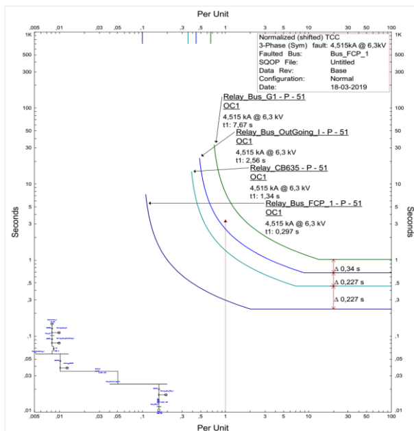
Gambar 5 Kurva Koordinasi Motor FCP 1
