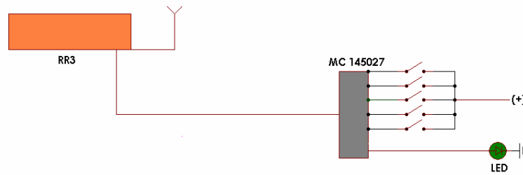
Figura 13: Esquema do Circuito Receptor do Ônibus. Fonte: Elaboração Própria.
