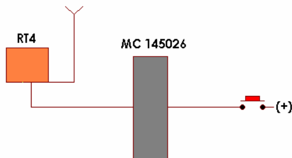
Figura 14: Esquema do Circuito Transmissor do Ônibus. Fonte: Elaboração Própria.
