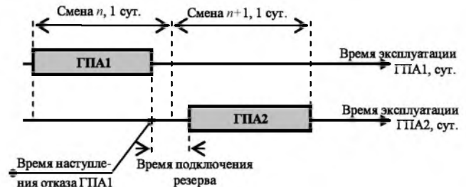
Рис. 4. Эксплуатация газокomppressorной установки в режиме отказа второго типа
