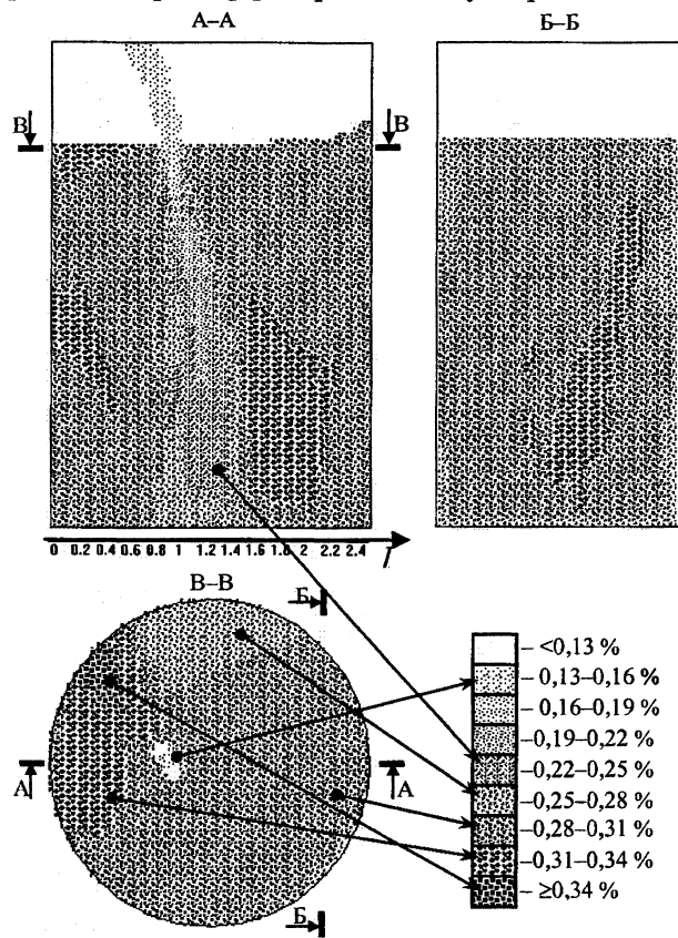
Рис. 3. Распределение концентрации углерода в различных сечениях ковша через 120 с после начала засыпки порошка
