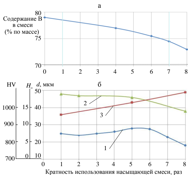
Рис. 5. Влияние кратности использования смеси на: а – содержание в ней бора; б – толщину (1); микротвердость боридного слоя на порошке ПР-Х18Н15 (2); твердость наплавленного слоя (3)
