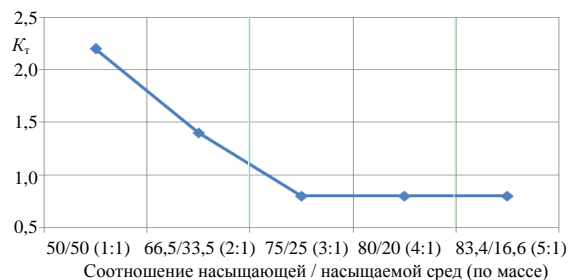
Рис. 2. Влияние соотношения компонентов в смеси на текучесть обработанного порошка ПР-Х18Н15: T = 920^\circ ; \tau = 2 ч
