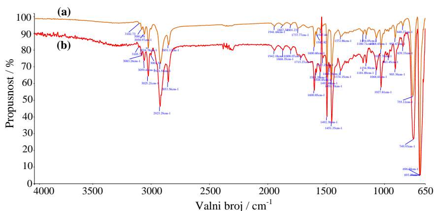
Slika 2. FTIR spektrogrami PS-E-a (a) i PS-E p -a (b).
