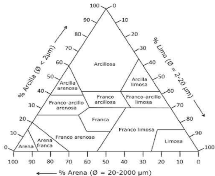
Figura 2. Diagrama para la determinación de la textura de un suelo.
