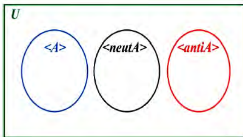
Fig. 5.1. Venn diagram
