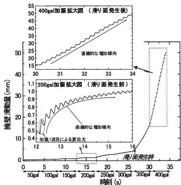
図1 重力式擁壁模型(水平支持層厚5cm)の滑動量
