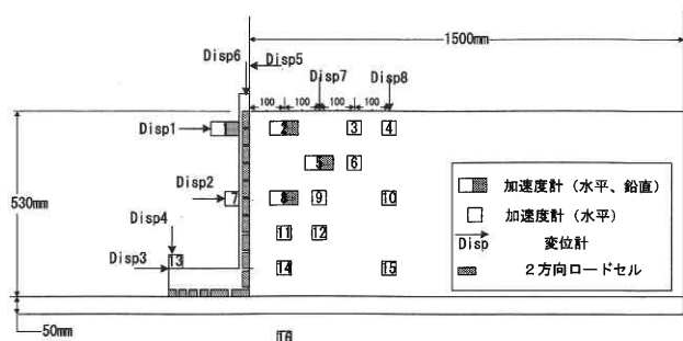
図2 重力式擁壁模型の断面図(水平支持層厚5cm)
