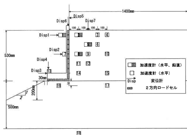
図5 重力式擁壁模型の断面図（斜面支持層厚50cm）
