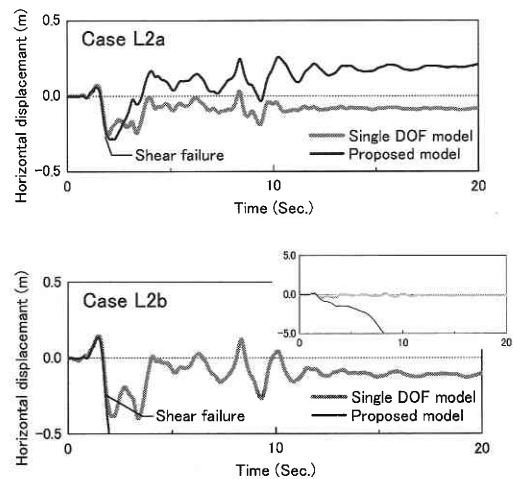
図 18 S39 橋脚の上端応答変位
