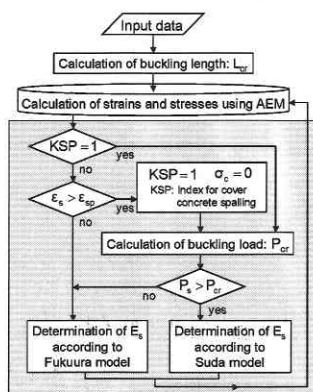
図7 提案モデルの解析フロー
