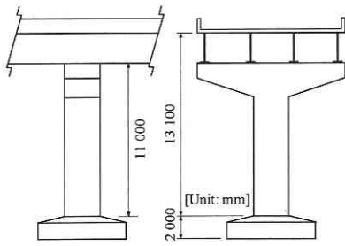
図 13 対象構造物
