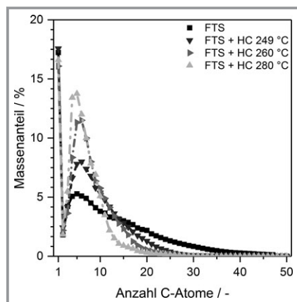
Abbildung 3. Einfluss der Temperatur der HC-Reaktion auf die Kohlenwasserstoffverteilung des zweistufigen Gesamtprozesses (FTS: 241 °C, 30 bar, H 2 /CO = 1,8, WHSV = 9,03 h -1 ), nach Sun [36].
