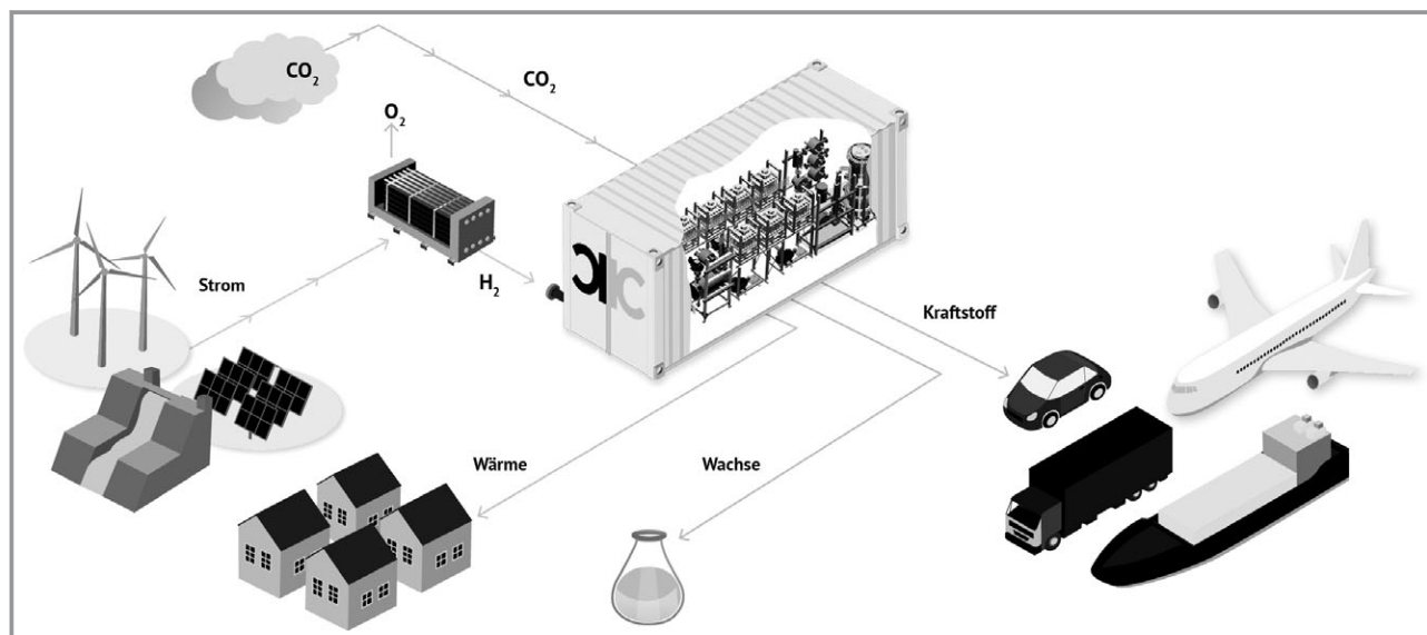
Abbildung 1. Power-to-Liquid-Prozess im Überblick. Aus Kohlenstoffdioxid und Wasser werden mithilfe von erneuerbarer Energie flüssige Kraftstoffe synthetisiert. Ein Weg der Wasserstoffbereitstellung ist die Elektrolyse. Die Abwärme der exothermen Synthese kann zum Beispiel zur Gebäudeheizung genutzt werden (Quelle INERATEC GmbH).
