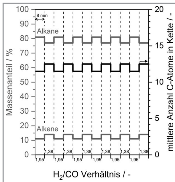
Abbildung 6. Lastwechselversuche in 8-Minuten-Intervallen. Ausgewählte Produkteigenschaften sind in Form von min-max-Bereichen über das Synthesegasverhältnis aufgetragen, das in den angegebenen Zeitintervallen eingestellt wurde.
