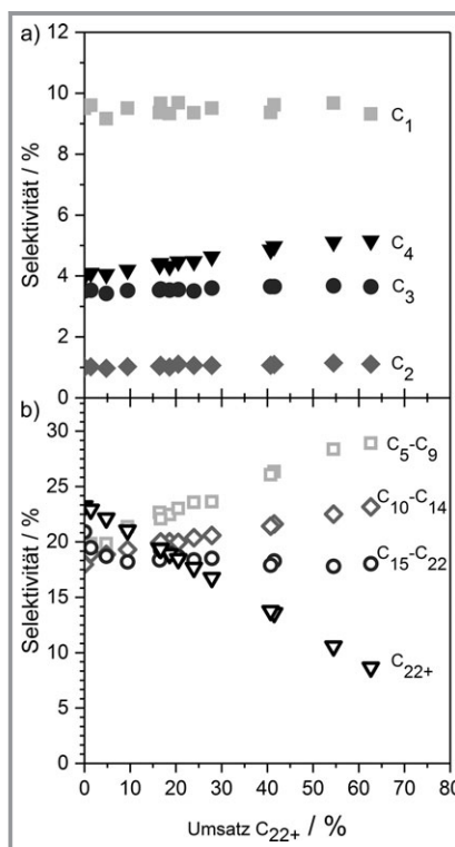
Abbildung 4. Integrale kohlenstoffnormierte Produktselektivitäten des Gesamtprozesses für verschiedene Wachsumsätze X C22+ im Hydrocracker bei konstantem FT-Zulauf. a) Gasförmige Produktfraktionen (FTS: X CO,FT = 50–52 %, 230 °C, 30 bar, H 2 /CO = 2, WHSV = 5,3 h -1 ; HC: 245–255 °C, WHSV = 21–63 h -1 , H 2 -Zudosierung: 0–3,2 L N min -1 ); b) flüssige bzw. feste Produktfraktionen.
