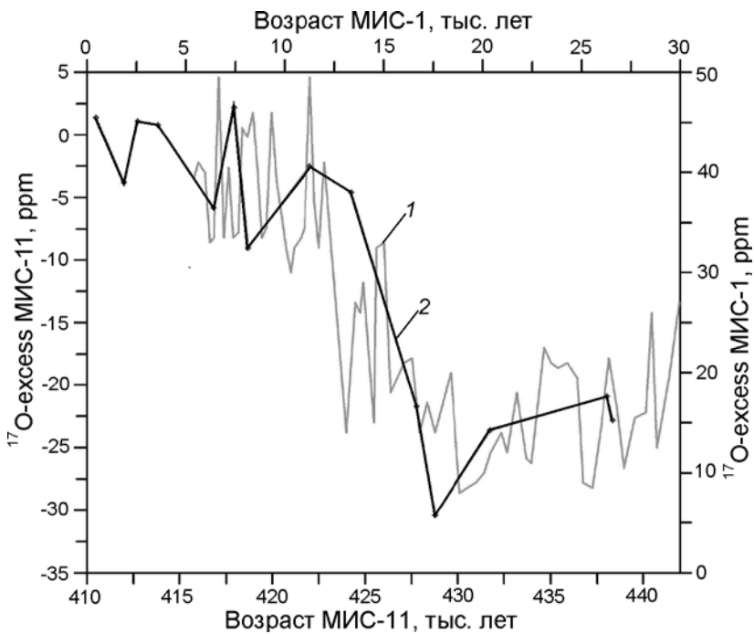
Рис. 3. Изменение ^{17}\text{O} -excess в интервалах керна станции Восток, соответствующих изотопным стадиям МИС-1 и МИС-11:
