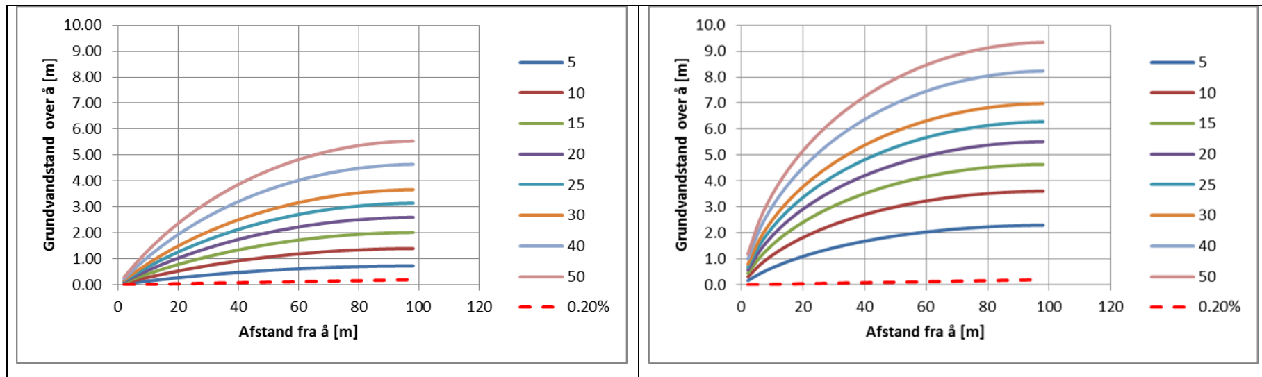
FIGUR 2.5. BEREGNEDE GRUNDVANDSPROFILER FOR JORDTYPEN JB5 PÅ MORÆNELER, PARAMETERISERET SOM VIST I TABEL 2.3. I VENSTRE KOLONNE ER D = 90M, I HØJRE KOLONNE ER D = 3 M.
