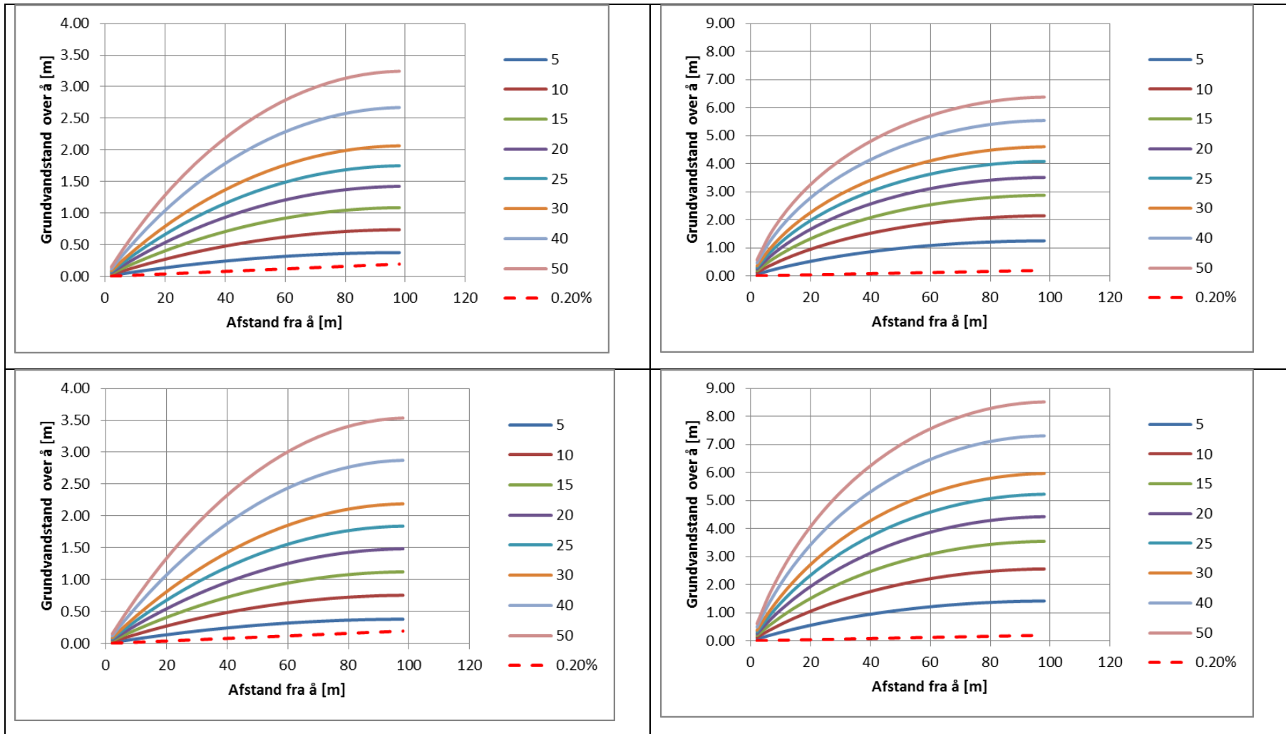
FIGUR 2.3. BEREGNEDE GRUNDVANDSPROFILER FOR JORDTYPERNE JB4 OG 5(OPPEFRA OG NED) PÅ TØRV, PARAMETERISERET MED EN HYDRAULISK LEDNINGSEVNE PÅ 17,3 M/DAG SOM VIST I TABEL 2.2. I VENSTRE KOLONNE ER DE = 20M, I HØJRE KOLONNE ER DE = 3 M.
