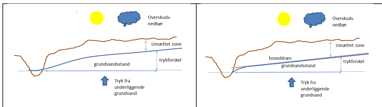
FIGUR 1. SKITSE TIL ILLUSTRATION AF GRUNDVANDETS BELIGGENHED I AFSTAND AF VANDLØBET, UDEN OG MED DRÆN INDLAGT.
