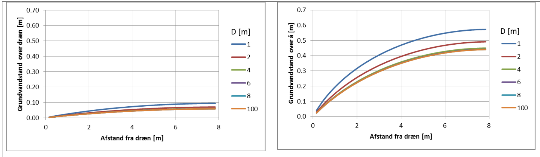
FIGUR 2.6. FORDELING AF GRUNDVANDSSTANDEN MELLEEM DRÆN LAGT MED 16 M'S AFSTAND BEREGNET MED PARAMETERISERINGEN BESKREVET I TABEL 2.3 FOR EN JB6 OG EN HYDRAULISK LEDNINGSEVNE I MORÆNELER PÅ 6,5 CM/DAG. TIL VENSTRE BEREGNET FOR EN GENNEMSITLIG AFSTRØMNING PÅ 5 MM/MÅNED, TIL HØJRE FOR 50 MM/MÅNED.
