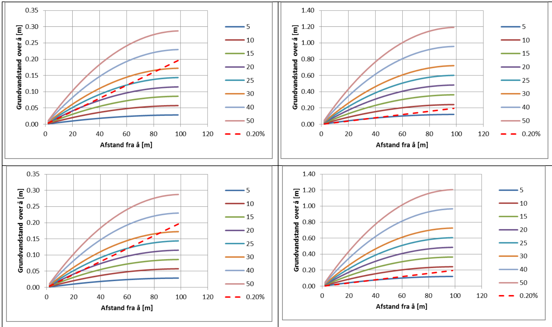
FIGUR 2.2. BEREGNEDE GRUNDVANDSPROFILER FOR JORDTYPERNE JB4 OG 5(OPPEFRA OG NED) PÅ TØRV, PARAMETERISERET MED EN HYDRAULISK LEDNINGSEVNE PÅ 232 M/DAG SOM VIST I TABEL 2.2. I VENSTRE KOLONNE ER DE = 20M, I HØJRE KOLONNE ER DE = 3 M.
