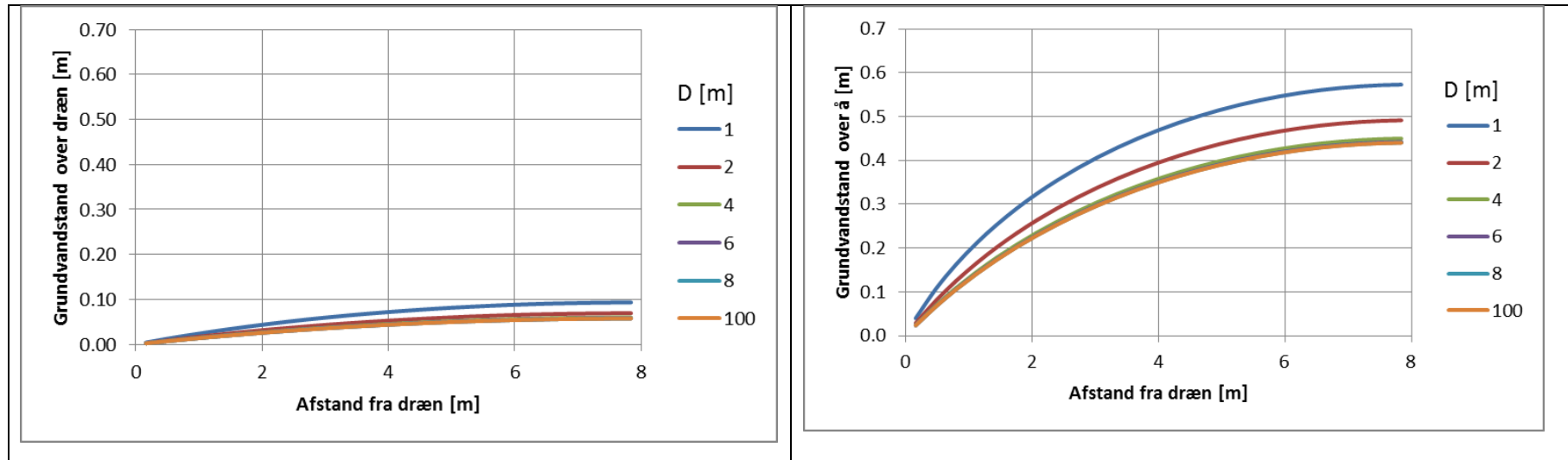
FIGUR 2.4. FORDELING AF GRUNDVANDSSTANDEN MELLEML DRÆN LAGT MED 16 M'S AFSTAND BEREGNET MED PARAMETERISERINGEN BESKREVET I TABEL 2.2 FOR EN JB5 OG EN HYDRAULISK LEDNINGSEVNE I TØRVEN PÅ 17.3 CM/DAG. TIL VENSTRE BEREGNET FOR EN GENNEMSITLIG AFSTRØMNING PÅ 5 MM/MÅNED, TIL HØJRE FOR 50 MM/MÅNED.
