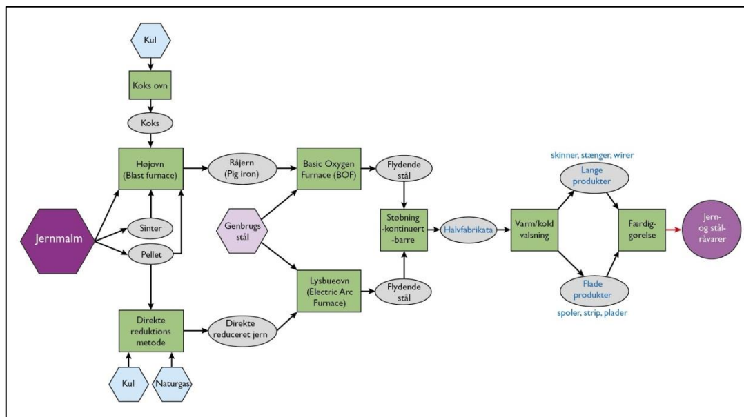
Figur 2-2. Oversigt over de procestrin og materialer, som er involveret, når jernmalm omdannes til jern- og stålprodukter (baseret på ERT 2013).
