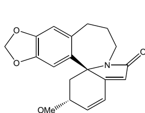
8-oxoschelhammeridine
