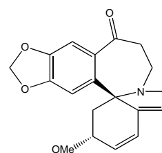
11a-oxoschelhammeridine
