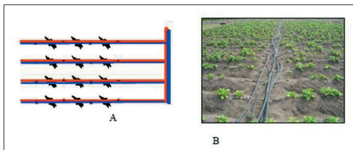
Drypslanger i kartoffelkamme for vandbesparende alternerende vanding. Ugentlig alterneres vandingstedet mellem den ene og den anden side af kartoffelplanten ved at vande enten gennem den blå eller den røde slange (A).
