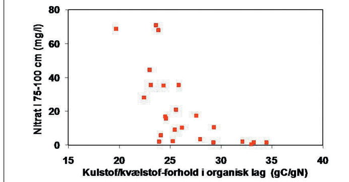
Figur 2. C/N-forholdet er en god indikator for nitratudvaskning fra skove. Når det falder til under 25, f.eks. som følge af luftforurening, øges koncentrationen af nitrat i det nedsivende vand.
