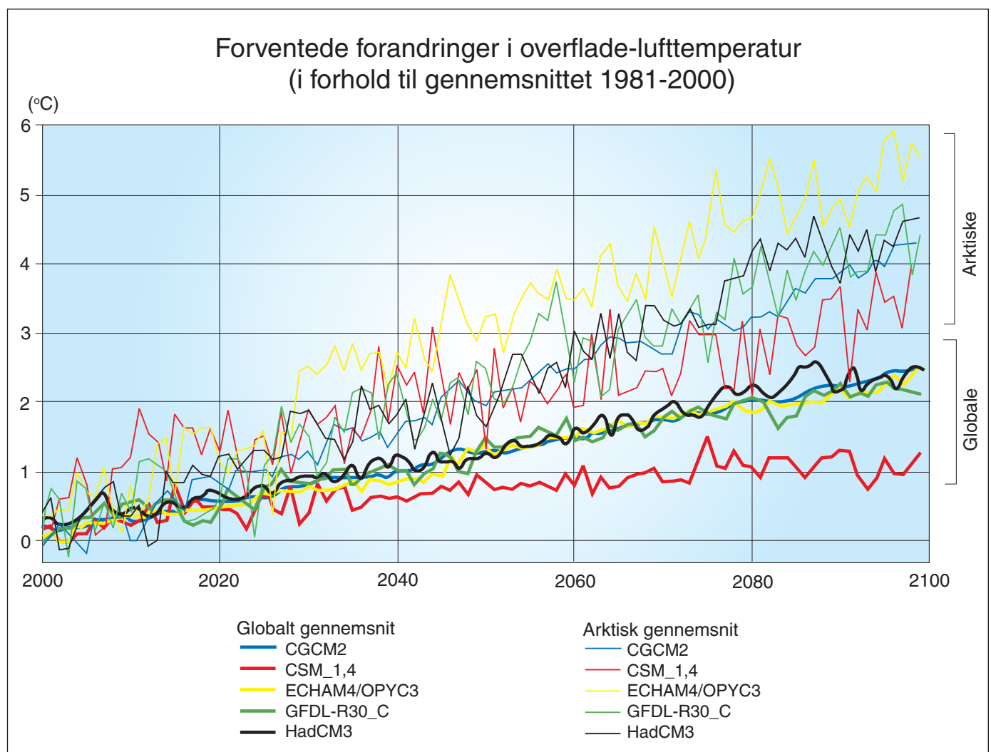
Temperaturudviklingen gennem det 21. århundrede ifølge 5 klimamodeller (generelle cirkulationsmodeller, GCMer) benyttet i Arctic Climate Impact Assessment-rapporten. De tykke streger er globalt midlede værdier, mens de tynde er arktiske middelværdier (60°-90°N). For alle modellerne ses det, at de forudsiger en væsentlig forstærket opvarmning på høje breddegrader. (Grafik: UVH modificeret efter ACIA-rapporten, http://www.acia.uaf.edu/ )
