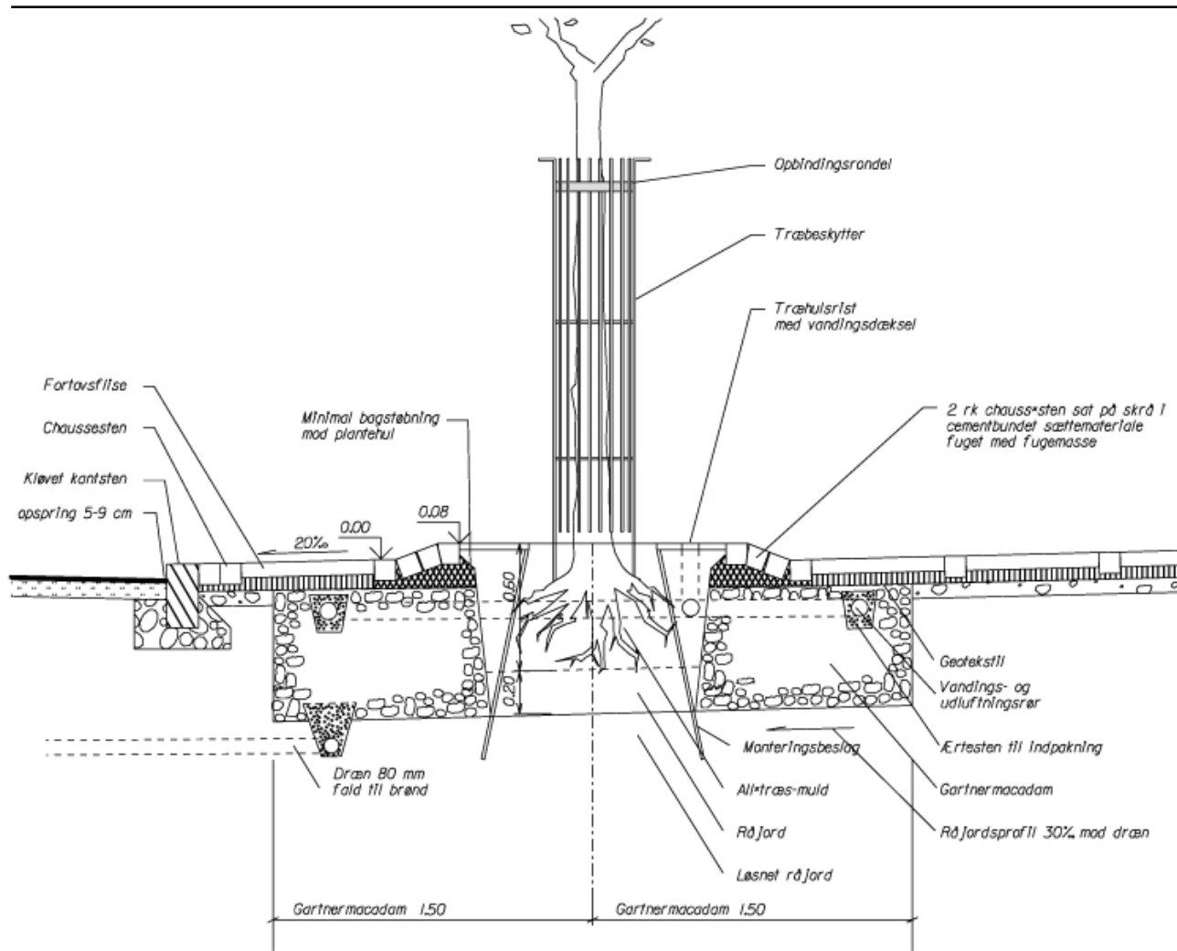
Figur 6: Principsnit af plantehul ved etablering med gartnermacadam.
