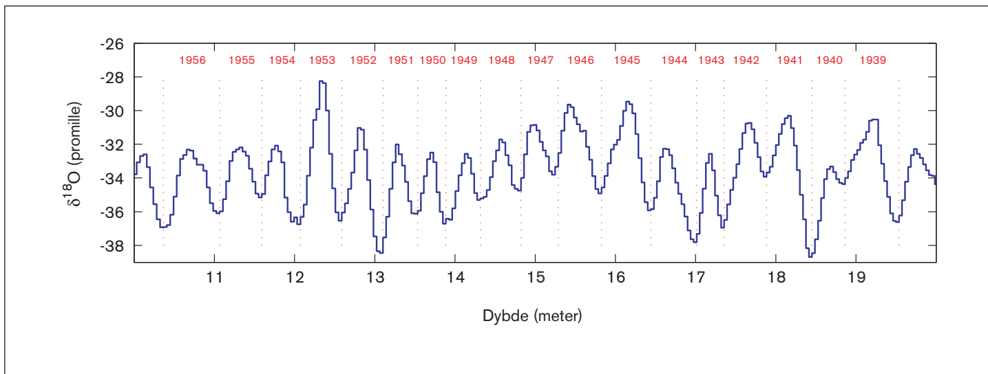
3. Den årlige temperaturvariation afspejles i isens isotopsammensætning, således at der er en større andel af de tunge isotoper, når der er varmt end når der er koldt (boks 2). Her ses isotopvariationen i 10 m iskerne fra Crête borestedet (fig. 2). Stykket indeholder omtrent 20 årlag, og en optælling af disse kan bruges til at datere isen med stor præcision.
