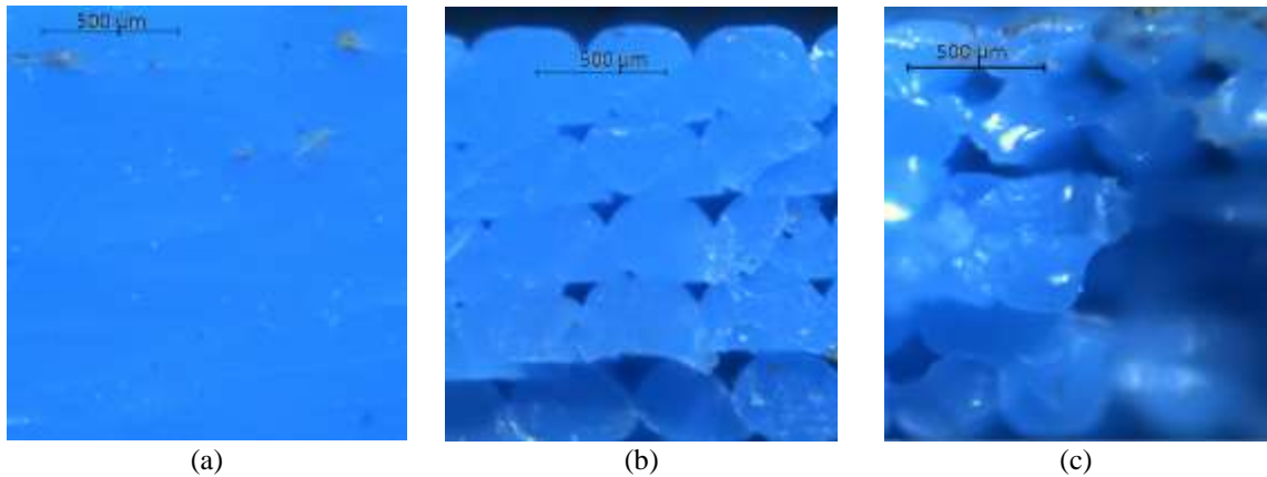
Figura 6: Macrográficas que muestran la superficie de fractura del material. (a) Sin ensayar; (b) Ensayado a 20 MPa; (c) Ensayado a 30 MPa. (50X)
