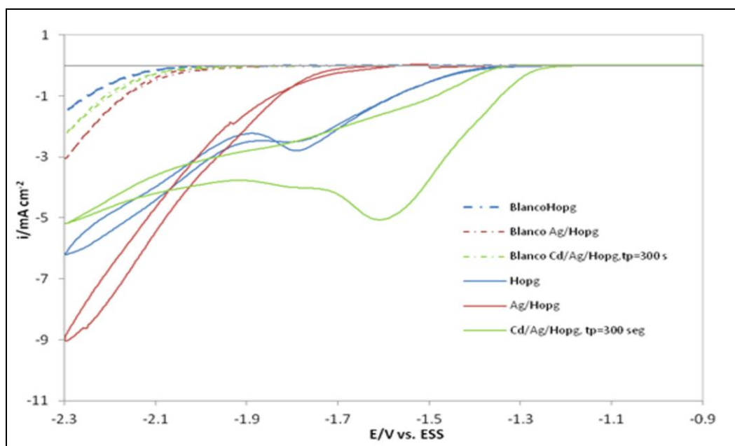
Figura 10: Comparación de la respuesta voltamperométrica de los sistemas: HOPG, Ag/HOPG, Cd-Ag/HOPG, en solución 0,1 M \text{Na}_2\text{SO}_4 y 0,1 M \text{NaNO}_3 + 0,1 M \text{Na}_2\text{SO}_4 , T=298 K, dE/dt=10 mV/s.
