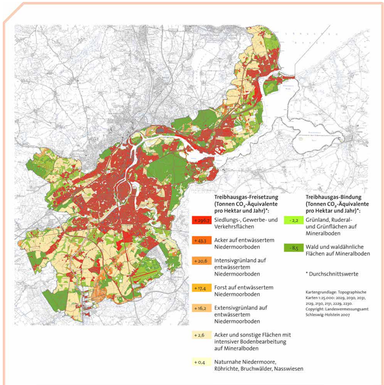
ABBILDUNG 9 – 6 ▶ ▶ Thematischer Landschaftsplan Lübeck, Entwurf: Treibhausgaswirksamkeit der aktuellen Landnutzungen.
