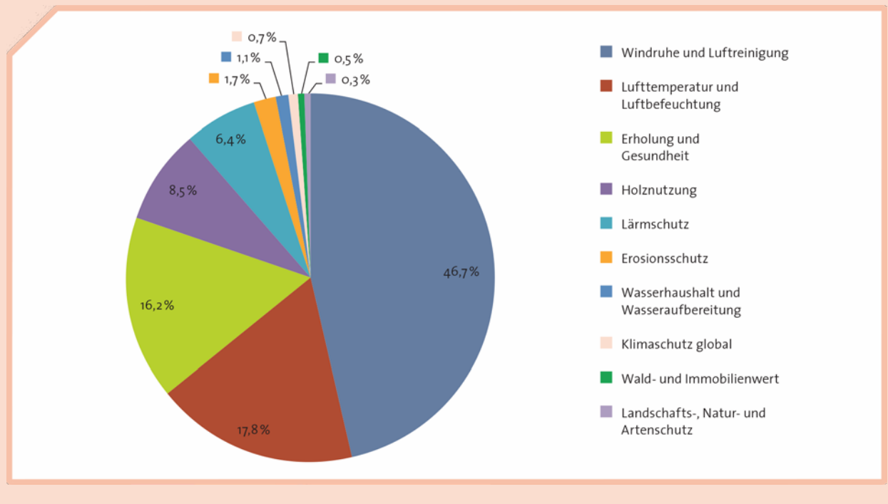
ABBILDUNG 7–8 ▶ Stadt Hagen: Volkswirtschaftlicher Wert der Ökosystemleistungen des Waldes im Stadtgebiet. Anteile in Prozent am Gesamtwert von 23 Mio. Euro pro Jahr. Waldfläche 6.900 Hektar. (Quelle: eigene Abbildung/Miriam Brenck nach Asche et al., 2015)
