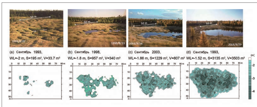
Процесс оттаивания вечной мерзлоты и рост озёр (Fedorov et al., 2014b)
