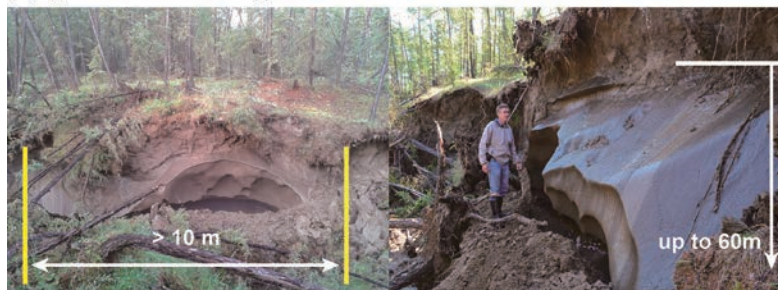
(а) Едома на абалахской террасе
