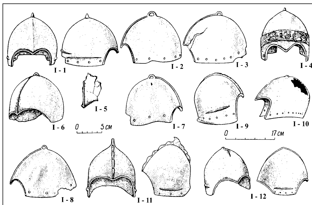
Fig. I. Cascos “Kuban”, según Galanina, 1985, Fig. 1. 1-2) Kelermes, kurgano 2 B. 3) Kelermes, kurgano 1 III. 4) Krymskaja, kurgano Voroncovskij. 5) Krymskaja, kurgano Macepinskij. 6) Gvardejskoe. 7) Sary Pečeur. 8-9) Lugar desconocido. 10) Siberia occidental. 11) Samarkanda. 12) Kysmyci.
