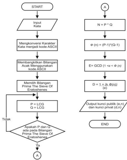
Gambar 5 Flowchart Pembangkit Kunci RSA
