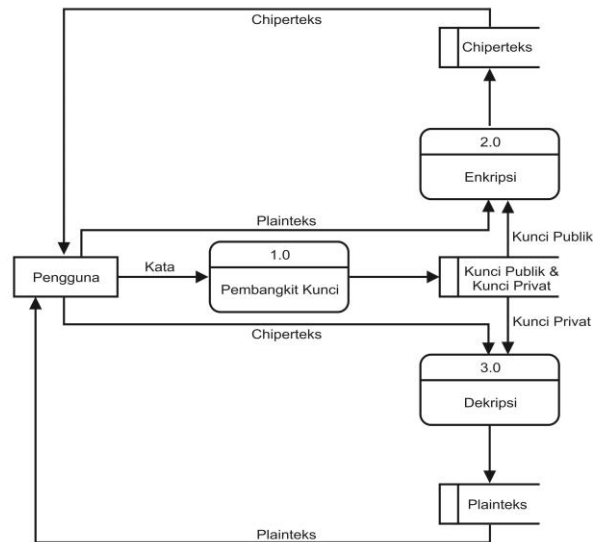
Gambar 4 Data Flow Diagram Aplikasi Kriptografi RSA
