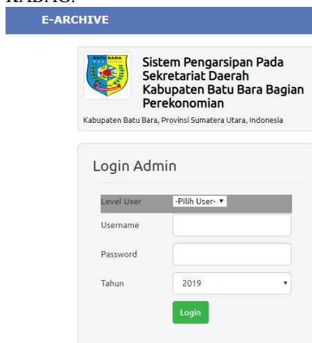
Fig. 8 Display Login
