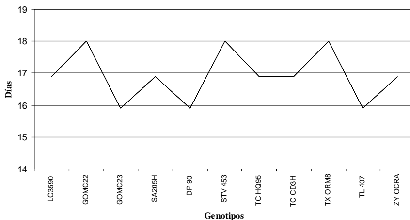
Figura 2. Tiempo de desarrollo del A. grandis en genotipos de algodón con diferentes características morfológicas, en Codazzi (Cesar, Colombia), 1996/97.
