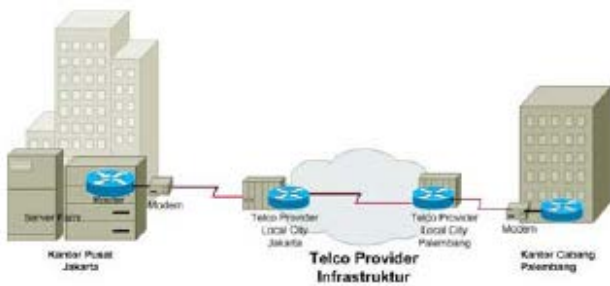
Gambar 1. Solusi Leased Channel Pada Jaringan Skala Luas (WAN)
