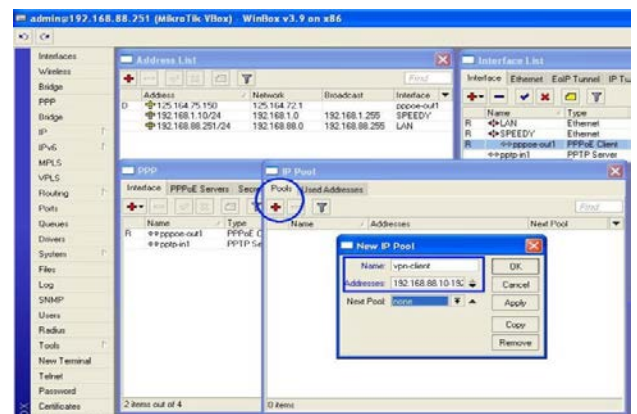
Gambar 10. VPN-Client
