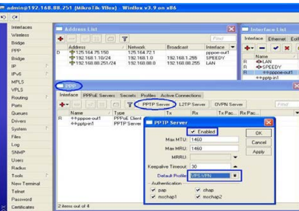
Gambar 13. Hasil Pembuatan PPTP Server
