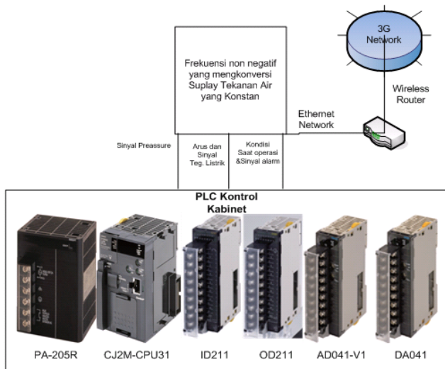
Gambar 6. Disain Data Akusisi
