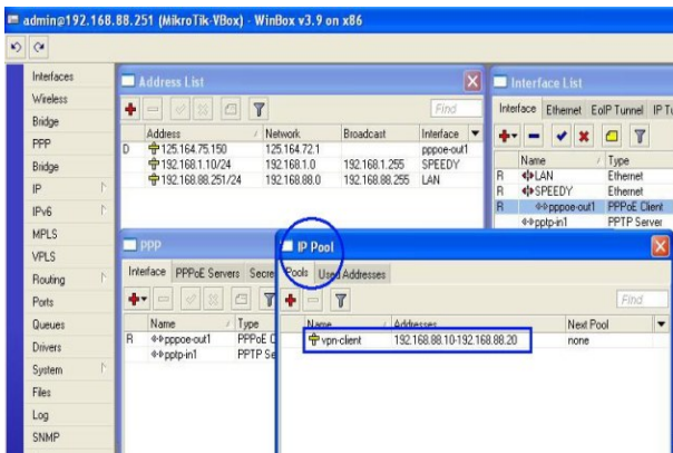
Gambar 11. Hasil pembuatan IPPool
