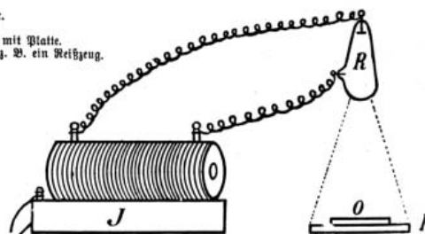
Ryc. 7. Obwód elektryczny lampy rentgenowskiej (baterie nie zostały pokazane) w niemieckiej broszurce z 1896 roku. J = izolator, R = lampa, K = klisza fotograficzna, O = przedmiot, który ma zostać prześwietlony za pomocą promieni X [13]
