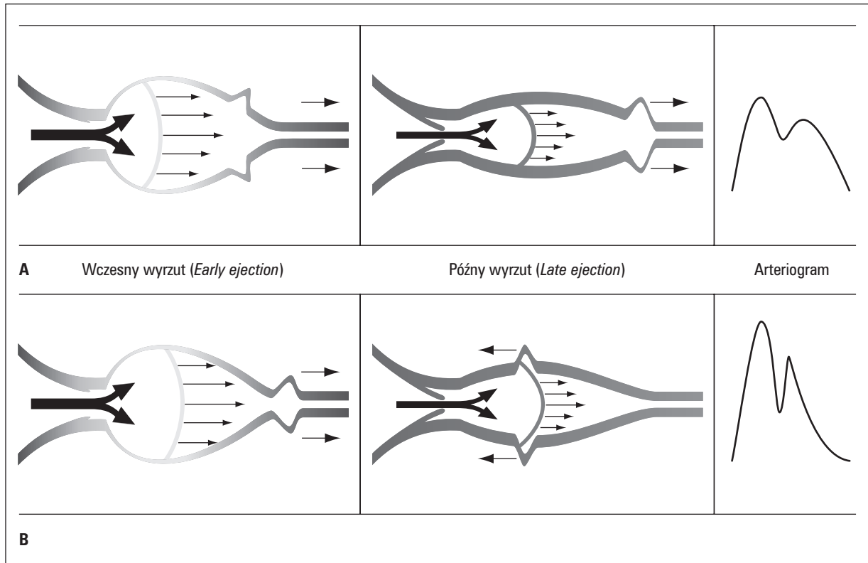
Rycina 11. Przebieg fali tętna w układzie tętniczym i powstawanie fali zwrotnej tętna. A. Prawidłowa ściana dużych tętnic o znacznej podatności. Pod koniec wyrzutu krwi z komory fala tętna odbita od dystalnych naczyń oporowych nie napotyka fali objętościowej krwi; B. Zmniejszona podatność dużych tętnic powoduje, że fala tętna rozprzestrzenia się szybciej. Fala odbita szybko wraca w kierunku serca i przed zakończeniem wyrzutu krwi do aorty interferuje z falą objętościową, powodując dodatkowe obciążenie następcze lewej komory serca i wzrost ciśnienia tętniczego
