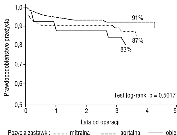
Rycina 1. Przyczyny zgonów (w nawiasach podano jedynie liczbę przypadków)
