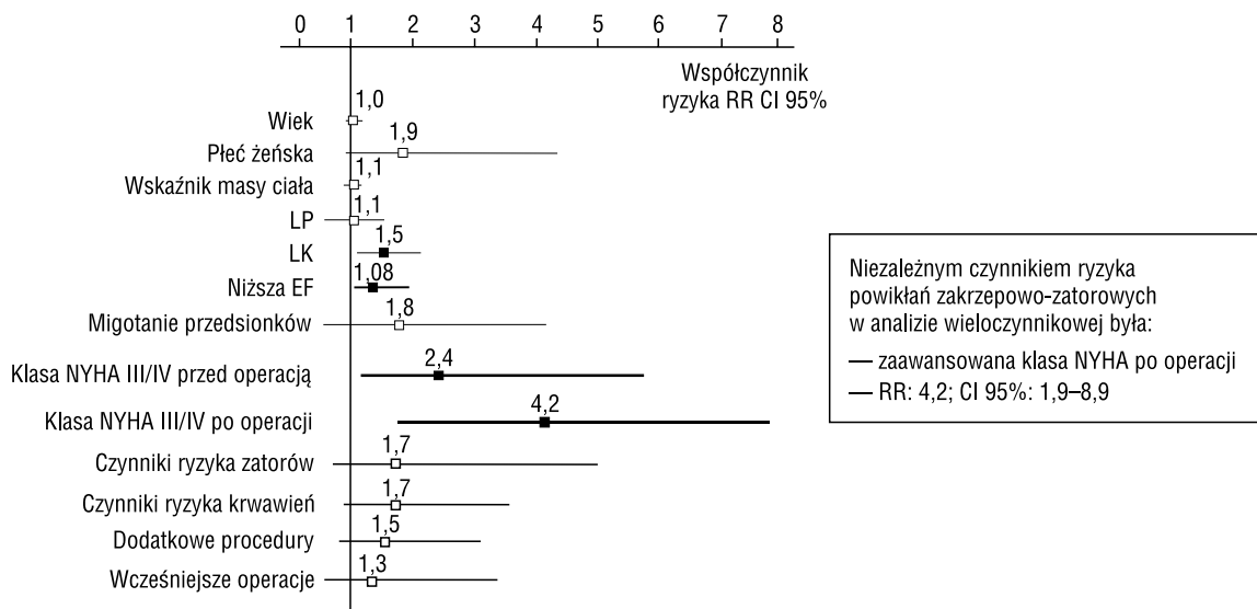
Rycina 3. Analiza jednoczynnikowa ryzyka powikłań zakrzepowo-zatorowych. LP — wielkość lewego przedsionka (RR określa wzrost ryzyka związany przyrostem wielkości przedsionka o 1 cm), LK — wielkość lewej komory (RR określa wzrost ryzyka związany z przyrostem wielkości lewej komory o 1 cm), EF ( ejection fraction ) — frakcja wyrzutowa lewej komory (RR określa wzrost ryzyka związany ze spadkiem EF o 1%, tu: spadek EF o 1% poniżej prawidłowej EF powoduje wzrost ryzyka o 8%). Czynniki ryzyka zatorów zdefiniowano jako tożsame z czynnikami ryzyka miażdżycy, np. nadciśnienie tętnicze, cukrzyca. Czynniki ryzyka krwawień zdefiniowano jako obecność chorób organicznych predysponujących miejscowo do krwawienia i występowanie krwawień w wywiadach.
