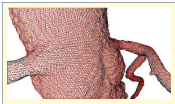
Rycina 4. Fragment aorty i początek tętnic wieńcowych po segmentacji, na który nałożono siatkę numeryczną. Przeprowadzenie obliczeń numerycznych na podstawie równania Naviera-Stokesa w poszczególnych komórkach obliczeniowych siatki umożliwia zobrazowanie rozkładu naprężeń ścinających działających na ścianę naczynia
