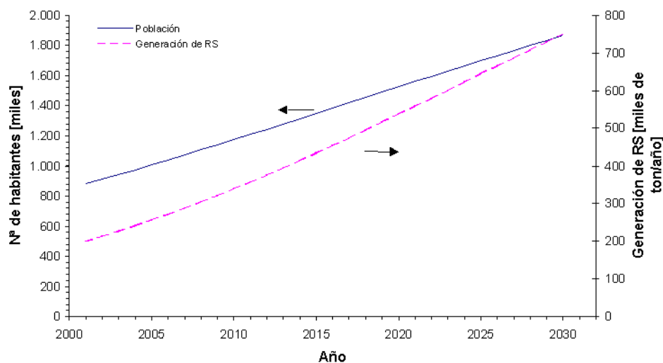
Figura 1: Proyecciones de la población y la generación anual de RS en la zona metropolitana de Cochabamba entre el 2000 y el 2030.
