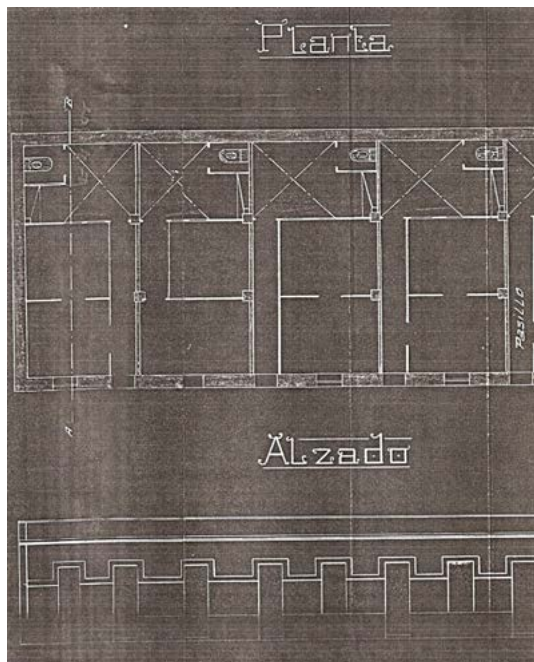
6. «Proyecto de construcción... de D. Emilio Gómez Gómez» (9 julio 1929). Arquitecto: Mauricio Jalvo —Planta por corte y alzado—.
