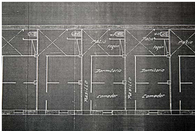
8. «Proyecto de construcción... de D. Emilio Gómez Gómez» (9 julio 1929). Arquitecto: Mauricio Jalvo —Planta—.
