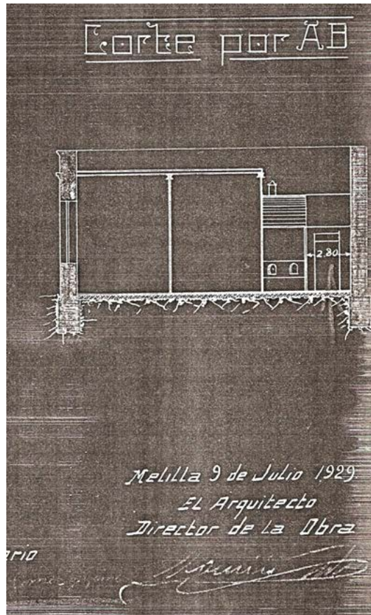
7. «Proyecto de construcción... de D. Emilio Gómez Gómez» (9 julio 1929). Arquitecto: Mauricio Jalvo —Corte por AB—.
