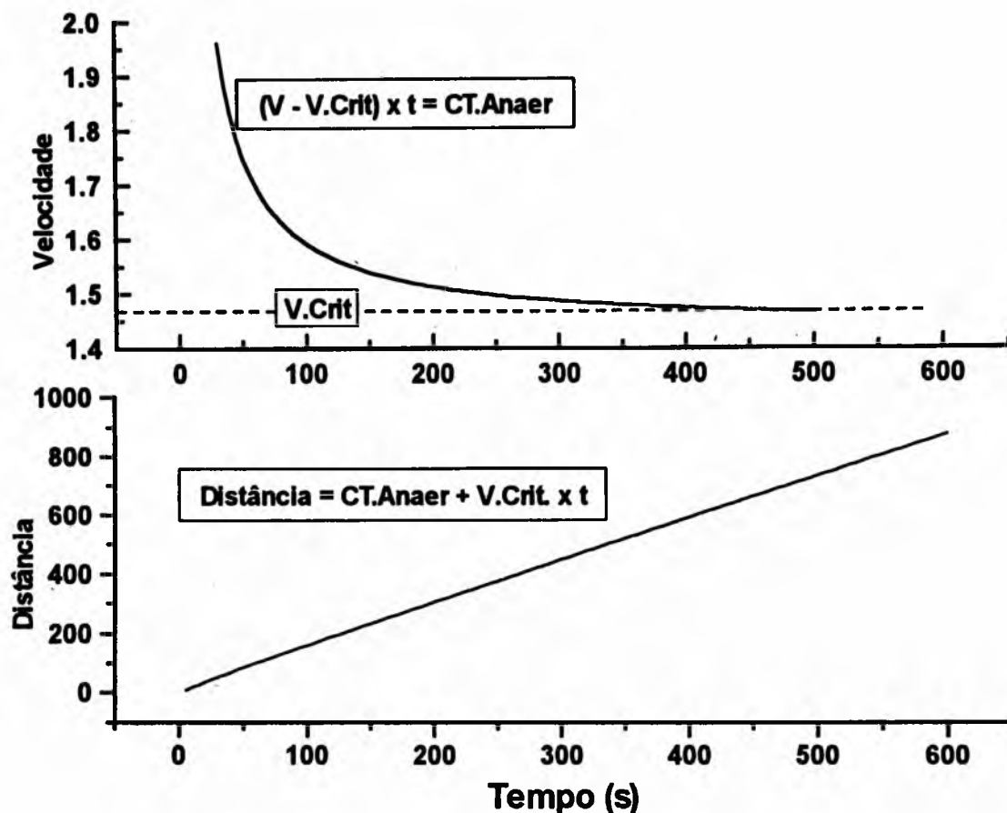
FIGURA 1 - Determinação da velocidade crítica segundo Overend et alii (1992). O gráfico à esquerda representa a função hipérbola entre velocidade e duração do esforço. À direita, a função linearizada, cuja inclinação, corresponde à velocidade crítica.
