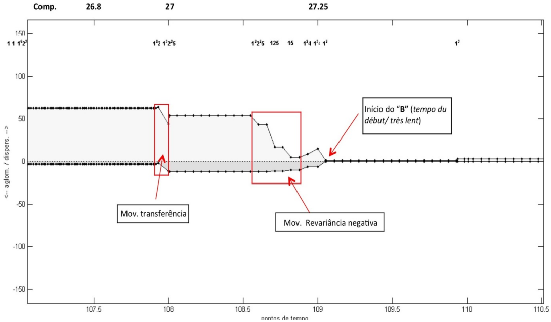
114 Figura 3: Indexograma de particionamento rítmico (pontos de tempo 107 a 110/ final da seção A) de Dérives 1 de Pierre Boulez. Gráfico gerado pelo programa Parsemat (GENTIL-NUNES, 2004).
