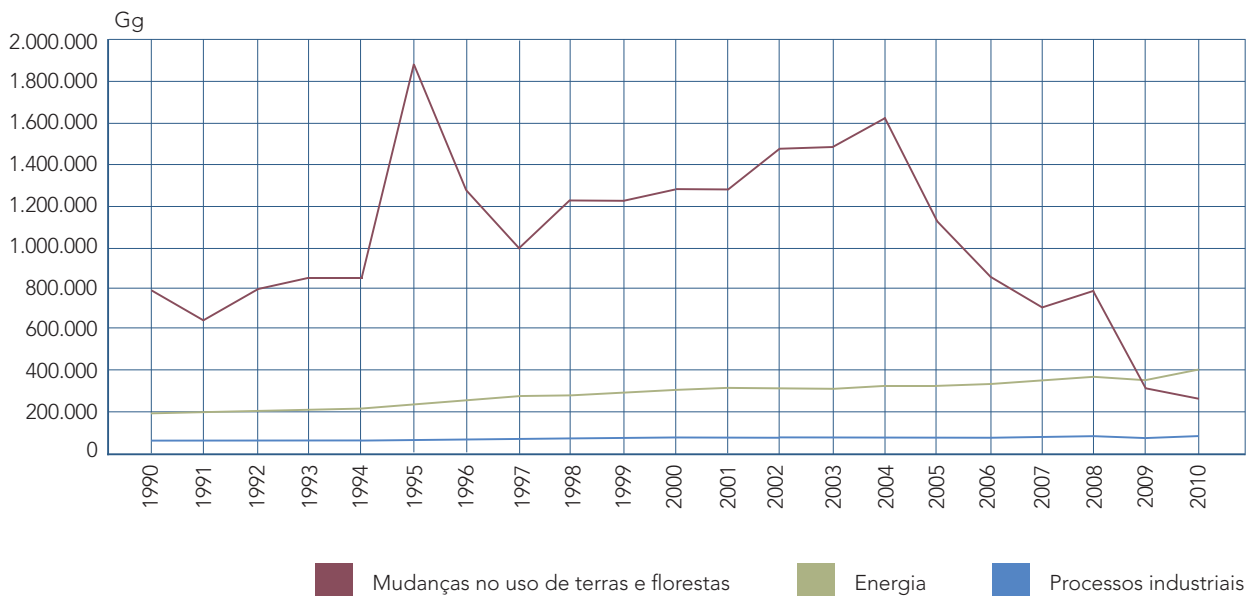
Gráfico 7 – Estimativas anuais de emissões de gás carbônico (CO 2 ), por setores de emissão, Brasil – 1990-2010. Fonte: Indicadores de Desenvolvimento Sustentável, Brasil, 2015. Instituto Brasileiro de Geografia e Estatística (IBGE)*
