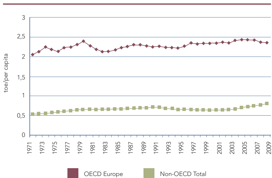
Gráfico 3 – Evolução do consumo final por habitante (1971-2009). Fonte: IEA, 2009. Energy Statistics.
