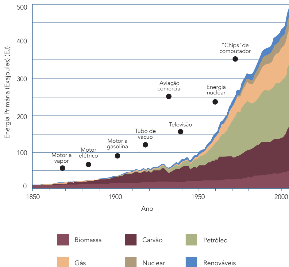
Gráfico 2 – A evolução do consumo mundial de energia (1850-2000). Fonte: GEA 2012 – Global Energy Assessment – Toward a Sustainable Future Cambridge University Press, Cambridge, UK.
