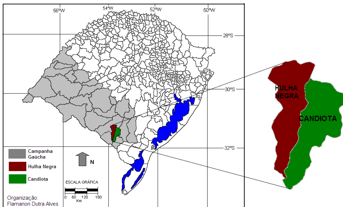
Figura 1 – Localização da região da Campanha Gaúcha e dos municípios de Candiota e Hulha Negra.
