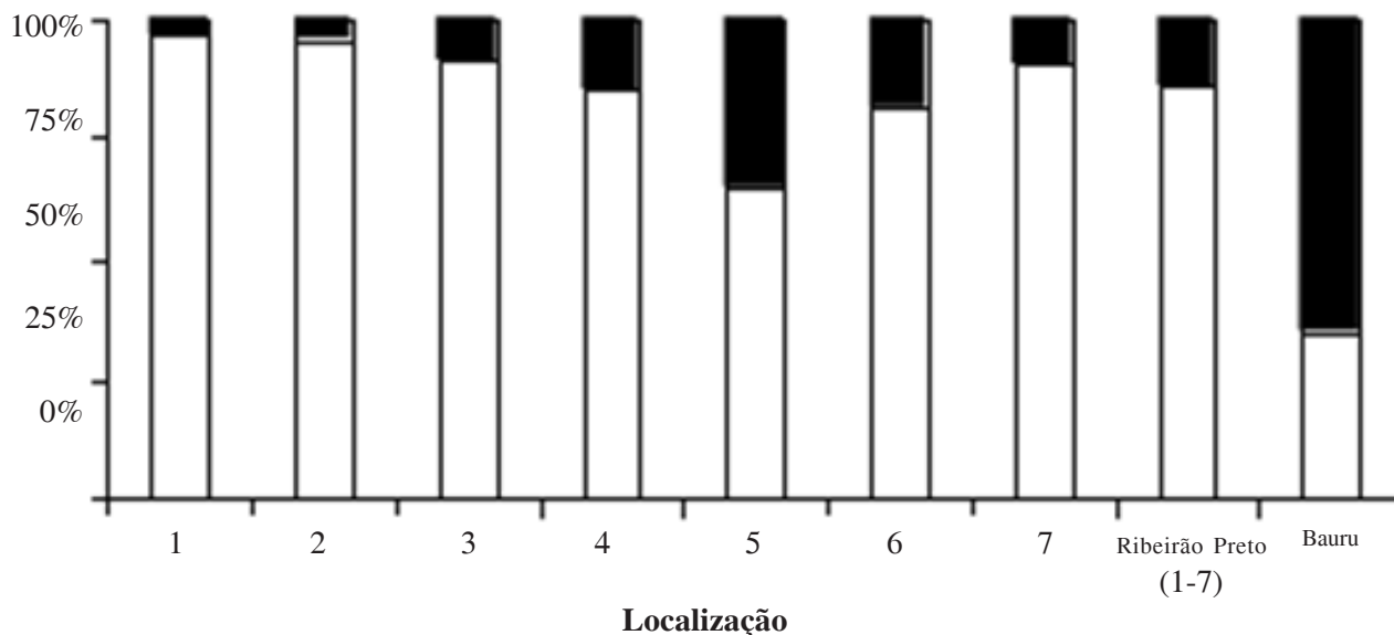
Figura 2. Porcentagens de crianças distribuídas de acordo com valores de chumbo 600 ou <600 \mu\text{g/g}</math> em amostras de esmalte superficial obtidas in vivo em 7 Escolas Municipais de Ribeirão Preto, SP ( n=186 ) e nas cercanias da Fábrica de Baterias AJAX, em Bauru, SP ( n=20 )(2004). Notar a maior porcentagem de crianças com chumbo de 600 \mu\text{g/g}</math> na Escola 5 de Ribeirão Preto em comparação com as demais. Figura reproduzida de Environmental Research 107: 264-70, 2008, com permissão da Editora Elsevier.
