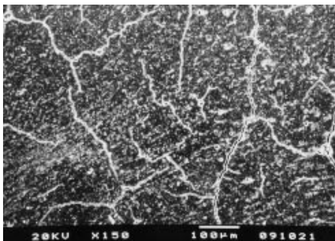
FIGURA 1 - Fotomicrografia do cimento de ionômero de vidro Vitremer. Grupo controle (150 X).
