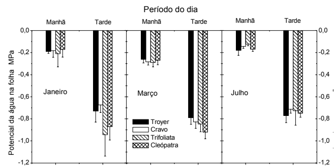
Figura 6 - Variação do potencial de água na folha em função do período do dia e do mês de medida em laranja 'Valência' sobre quatro espécies de porta-enxerto. Barras indicam desvio padrão da média. Campinas, 1998.
