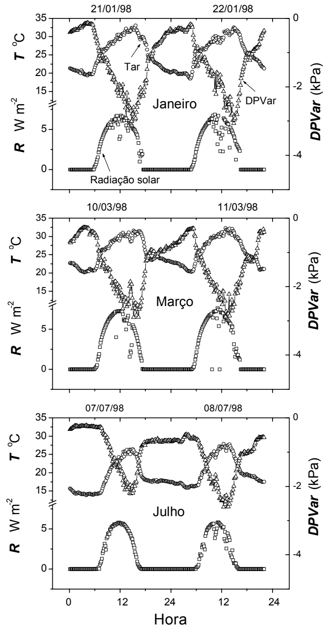
Figura 1 - Variação da temperatura do ar ( T ), da radiação solar ( R ) e do déficit de pressão de vapor do ar ( DPV_{ar} ) nos dias de medidas de trocas gasosas em laranja 'Valência' sobre quatro espécies de porta-enxerto. Campinas, 1998.
