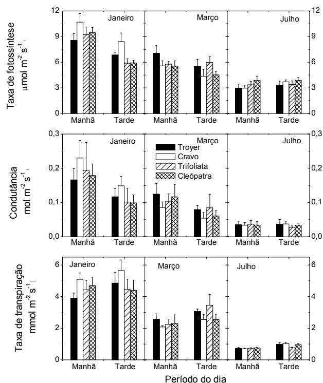
Figura 2 - Variação da taxa de fotossíntese, da condutância estomática e da transpiração em função do período do dia e do mês de medida em laranja 'Valência' sobre quatro espécies de porta-enxerto. Barras indicam desvio padrão da média. Campinas, 1998.
