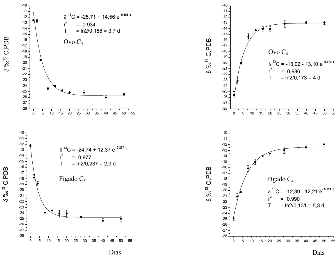
Figura 2 - Modelo exponencial para os isótopos estáveis do carbono (média + desvio padrão, n = 3) em ovo e fígado de aves de postura adultas alimentadas com dietas formuladas à base de plantas dos ciclos fotossintéticos C 3 e C 4 . Carrijo (2000).
